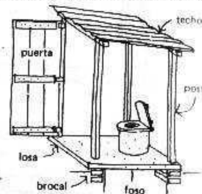
Vista en corte de una letrina.
