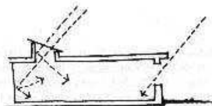
techo plano: tragaluz
