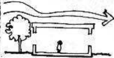
árboles bajos: la brisa sube y no entra
