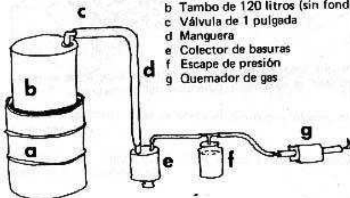
las partes de un tambo-digestor
