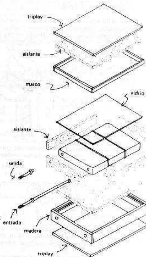
las partes de un calentador de 40 litros
