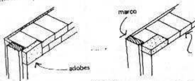
Maneras de proteger las esquinas, reforzándolas.
