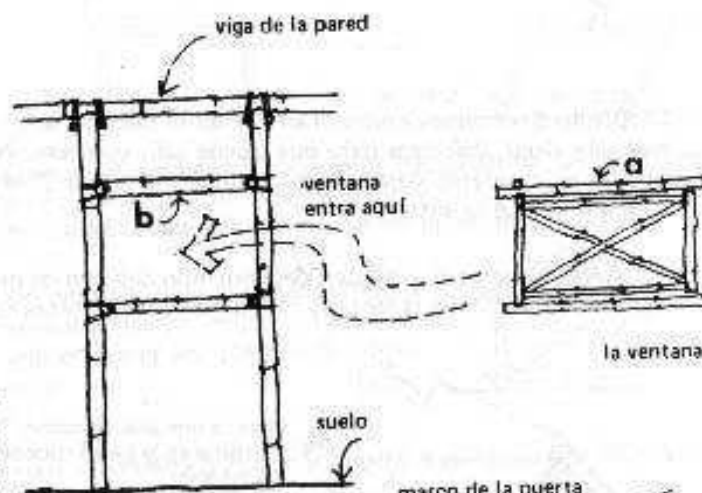
Marco de la ventana
