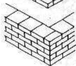
Cruce de hiladas en esquinas
