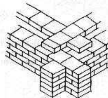
Las hiladas se cruzan, y sobresale el ancho de un adobe
