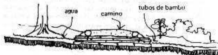
corte de una alcantarilla
